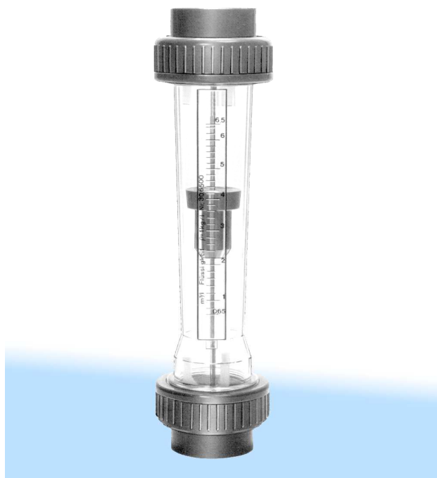
Fig. 1 Débitmètre à flotteur F VA Trogflux
